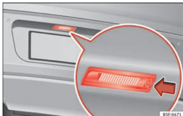
Abb. 115 Im Stoßfänger hinten: Kennzeichenbeleuchtung.
