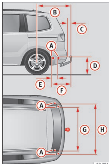
Abb. 231 Maße und Befestigungspunkte zum Nachrüsten einer Anhängervorrichtung.
