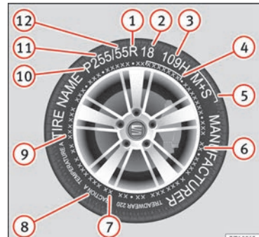
Abb. 253 Internationale Reifenbeschriftung.
