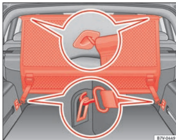
Abb. 167 Im Gepäckraum: Netztrennwand hinter der zweiten Sitzreihe einbauen
