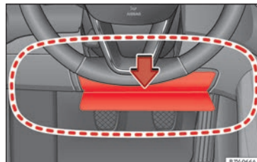
Abb. 29 Auf der Fahrerseite: Wirkungsbereich des Knieairbags.
