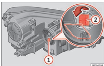
Abb. 108 Blinklichtlampenhalter (1) und Abbiegelicht (2).
