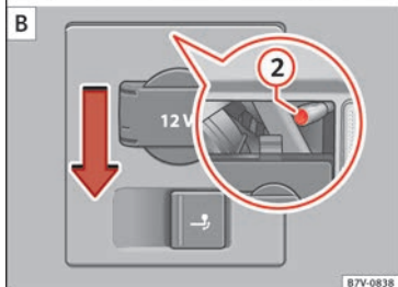
Abb. 113 Im Seitenbereich des Gepäckraums: linke und rechte Rückleuchten ausbauen. ① Abdeckkappe abziehen, ② Befestigungsschraube.
