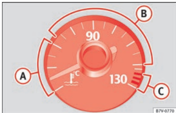
Abb. 243 Motorkühlmitteltemperaturanzeige im Kombiinstrument: A Kaltbereich; B Normalbereich; C Warnbereich.
