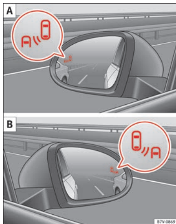
Abb. 220 In den Außenspiegeln: Anzeige des Blind-Spot-Assistenten.
