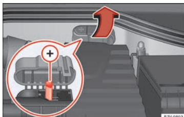
Abb. 74 Im Motorraum: Starthilfe Pluspol (+).
