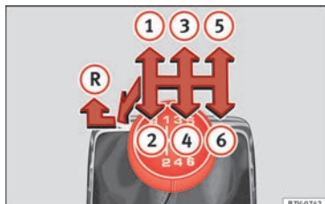
Abb. 47 Schaltschema des 6-Gang-Schaltgetriebes.
