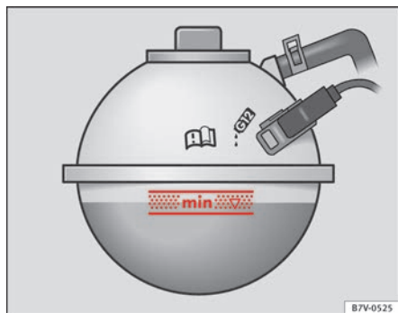
Abb. 171 Im Motorraum: Markierung an dem Motorkühlmittelausgleichsbehälter.
