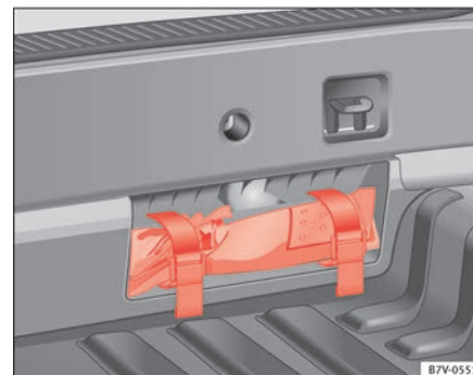
Abb. 197 Im Gepäckraum vom Fahrzeuginnenraum aus gesehen: Bordwerkzeug in einer Mulde im Bereich des Schlossträgers.
