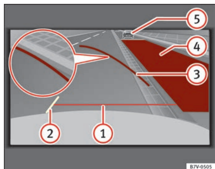
Abb. 149 Im Bildschirm: Orientierungslinien und -flächen des Parkraums hinter dem Fahrzeug.
