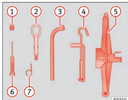
Abb. 198 Bestandteile des Bordwerkzeugs.
