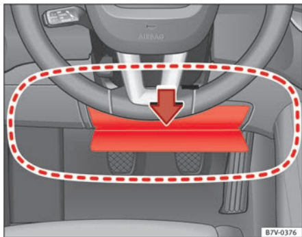
Abb. 25 Auf der Fahrerseite: Wirkungsbereich des Knieairbags.
