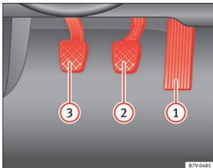
Abb. 128 Pedale bei Fahrzeugen mit Schaltgetriebe: ① Gaspedal, ② Bremspedal, ③ Kupplungspedal.
