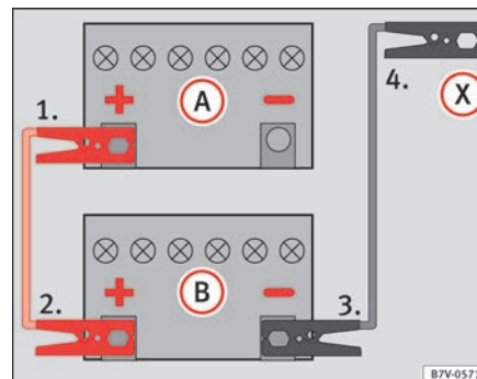
Abb. 216 Schema für das Anklemmen der Starthilfekabel bei Starthilfer-Fahrzeugen ohne Start-Stopp-Betrieb: entladene Fahrzeugbatterie (A) und Strom gebende Fahrzeugbatterie (B).
