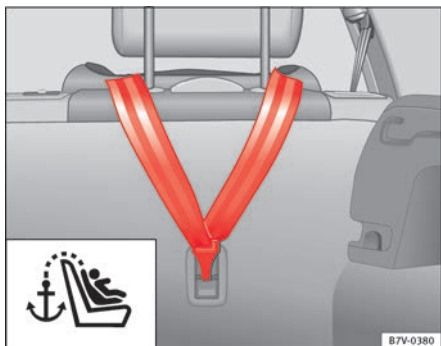
Abb. 28 Eingehängter oberer Befestigungsgurt im Gepäckraum.
