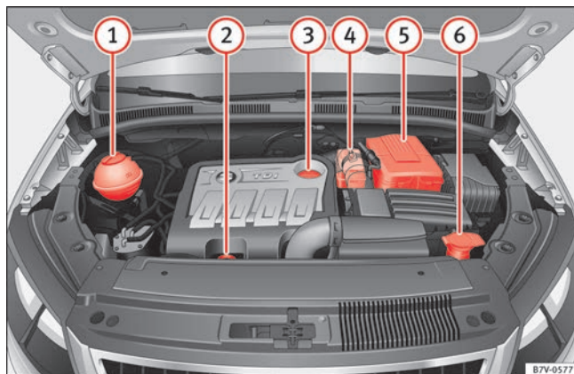
Abb. 221 Abbildung für die Einbaustellen der Elemente
