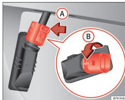
Abb. 214 Kennzeichenleuchte: Lampenhalter ausbauen.
