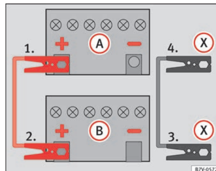
Abb. 217 Schema für das Anklemmen der Starthilfekabel bei Starthilfer-Fahrzeugen mit Start-Stopp-Betrieb: entladene Fahrzeugbatterie (A) und Strom gebende Fahrzeugbatterie (B).
