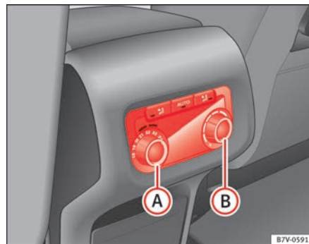
Abb. 123 Detailansicht der Fondbedienung
