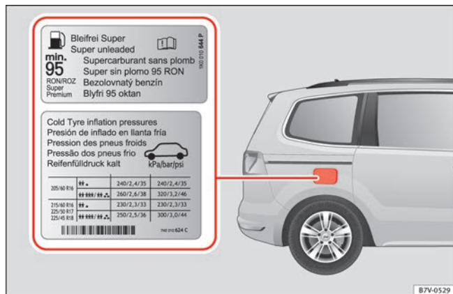
Abb. 176 Einbauort des Reifenfülldruckschildes.
