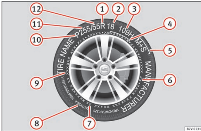
Abb. 178 Internationale Reifenbeschriftung.
