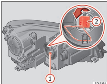
Abb. 206 Blinklichtlamphenhalter (1) und Abbiegelicht (2).
