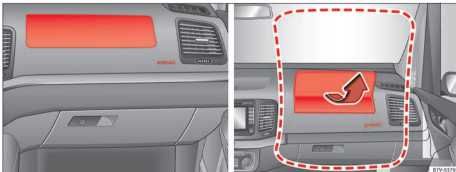
Abb. 18 Einbauort und Wirkungsbereich des Beifahrer-Frontairbags.
