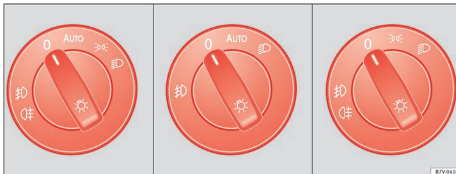
Abb. 62 Neben dem Lenkrad: Darstellung einiger Varianten des Lichtschalters.
