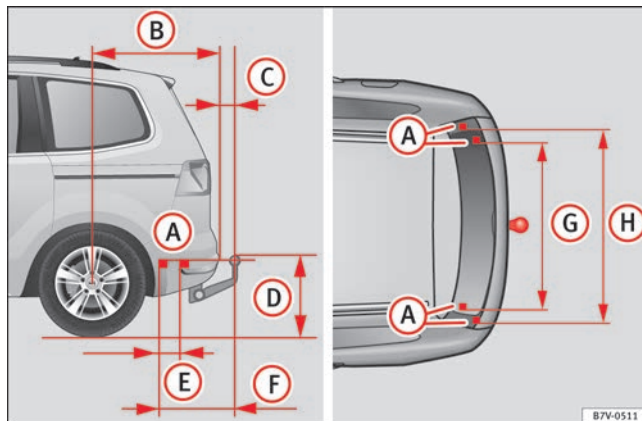
Abb. 157 Maße und Befestigungspunkte zum Nachrüsten einer Anhängervorrichtung.
