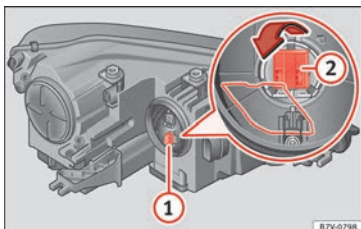
Abb. 108 Blinklichtlampenhalter (1) und Abriegellicht (2).
