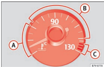
Abb. 245 Motorkühlmitteltemperaturanzeige im Kombiinstrument: A Kaltbereich; B Normalbereich; C Warnbereich.
