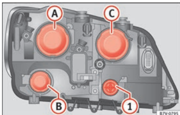
Abb. 105 Im Motorraum: Verkleidungen im linken Scheinwerfer. A Abblendlicht, B Tagfahrlicht und C Fernlicht und Standlicht.
