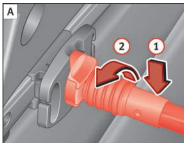
Abb. 171 Kuvertnetz aushängen.
