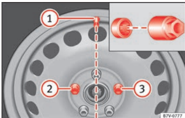
Abb. 68 Radwechsel: Reifenventil ① und Einbauort der Anti-Diebstahl-Radschraube ② oder ③.
