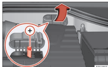
Abb. 74 Im Motorraum: Starthilfe Pluspol (+).
