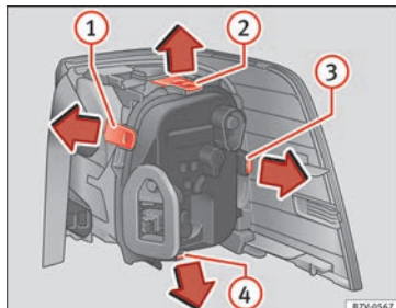
Abb. 114 Rückleuchte in der Karosserie: Lampenträger ausbauen. ① bis ④ Verriegelungslaschen.
