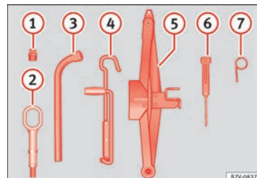
Abb. 64 Im Gepäckraum unter dem Gepäckraumboden: Bordwerkzeug.
