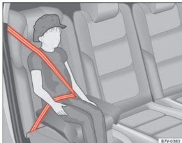
Abb. 95 Integrierter Kindersitz: Gurtbandverlauf.
