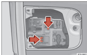
Abb. 112 In der Heckklappe: Lampenträger herausnehmen.
