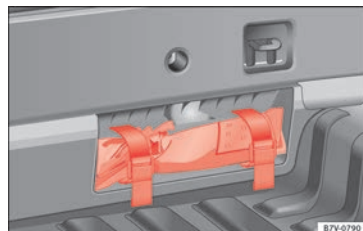
Abb. 99 Im Gepäckraum, vom Fahrzeuginnenraum aus gesehen: Bordwerkzeug in einem Hohlraum im Bereich des Schlossträgers.
