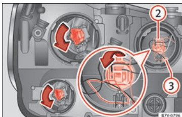
Abb. 106 Linker Scheinwerfer.
