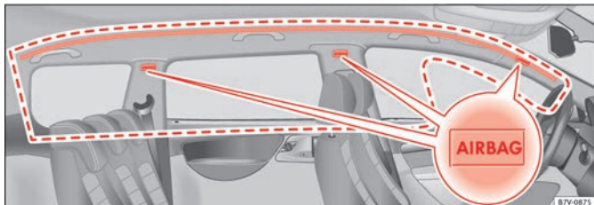
Abb. 32 An der linken Fahrzeugseite: Einbauort und Wirkungsbereich des Kopfairbags. »»
