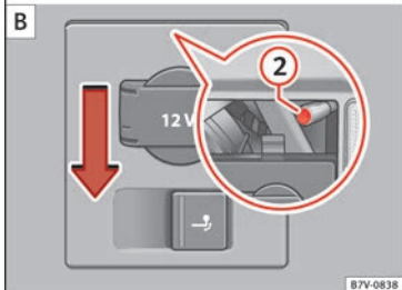
Abb. 113 Im Seitenbereich des Gepäckraums: linke und rechte Rückleuchten austauschen. ① Abdeckkappe abziehen, ② Befestigungsschraube.
