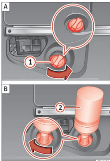
Abb. 239 AdBlue-Tank mit Verschluss des Tankeinfüllstutzens und Nachfüllflasche.
