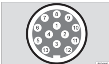
Abb. 232 Schematische Darstellung: Zuweisung der Steckverbinderstifte für Anhängerstrom.
