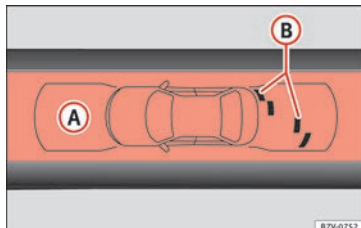
Abb. 211 Anzeige im Display des OPS: A Hindernis im Segment erkannt; B Abgetasteter Bereich vor dem Fahrzeug.
