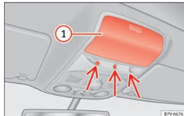
Abb. 133 In der Dachkonsole: Sensoren der Innenraumüberwachung.
